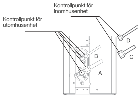
A: Lågtrycksventil B: Högtrycksventil C & D: Flänsmuttrar till inomhusenhet
