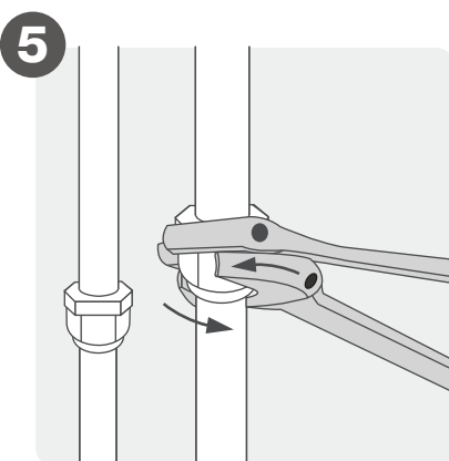
Anslut rören
